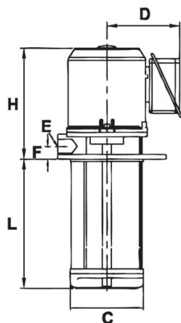
此為JW-4 (1/4HP)規格
