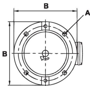
此為JW-4 (1/4HP)規格
