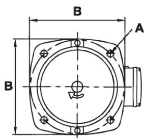
此為JW-8 (1/8HP)規格
